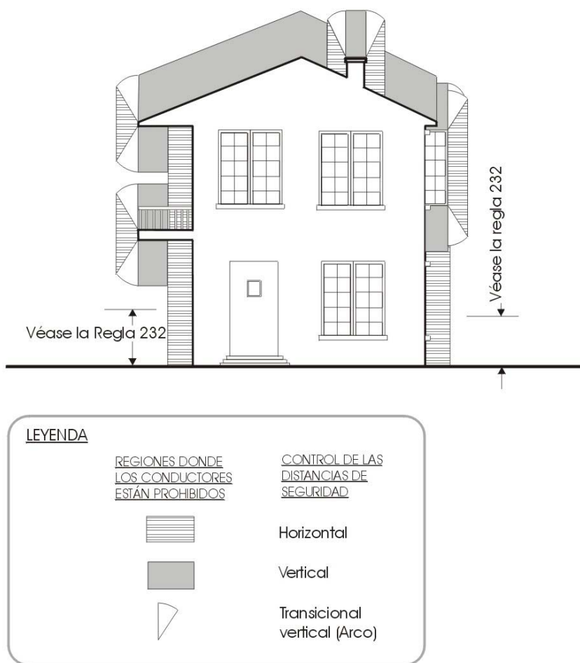
Figura 234-1 (a) DIAGRAMA DE LA DISTANCIA DE SEGURIDAD PARA UNA EDIFICACIÓN
