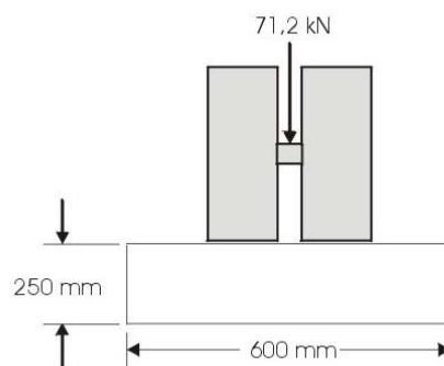
Figura 223-2 ÁREA DE CARGA DE LAS RUEDAS
