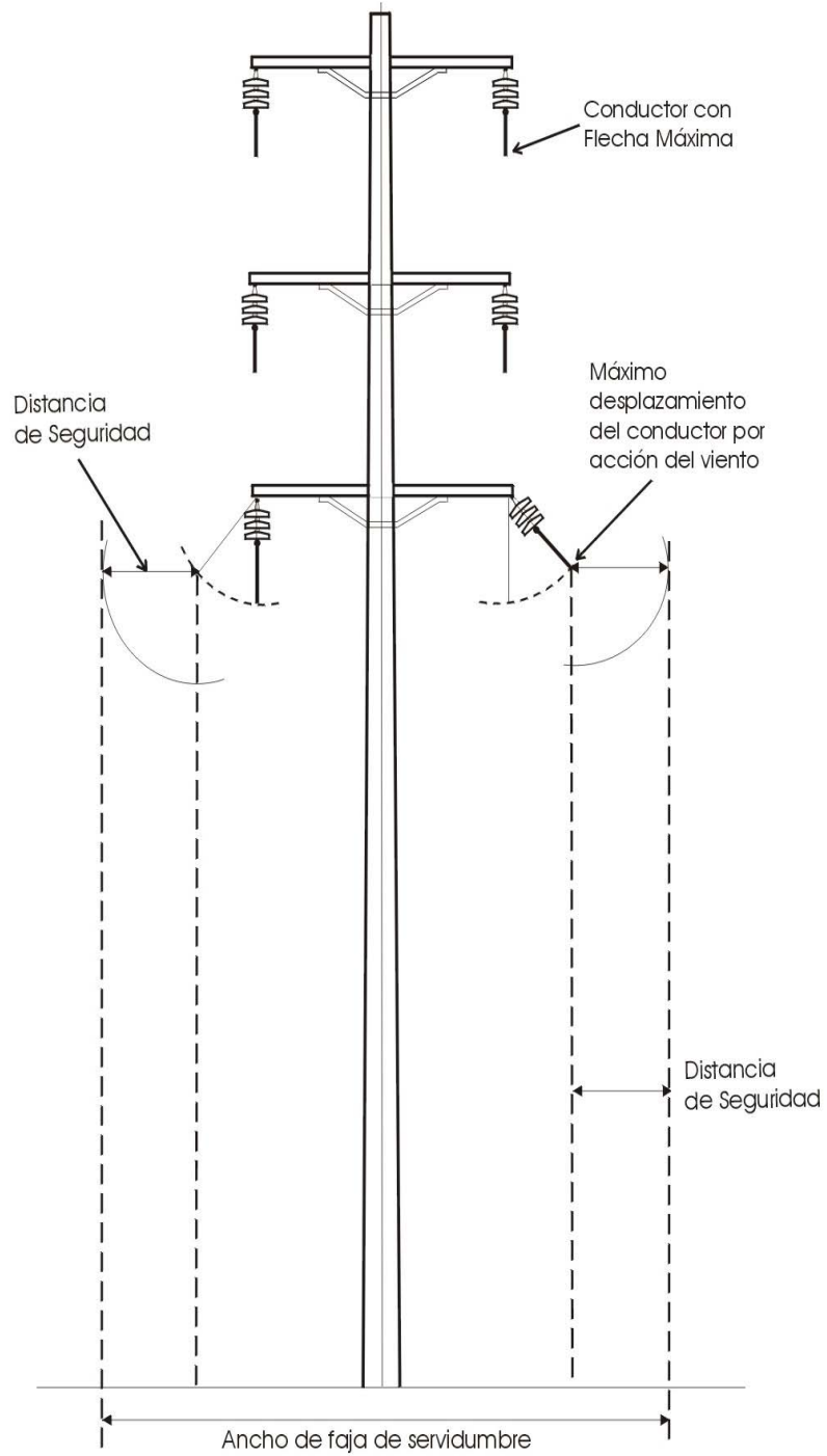
Figura 219 FAJA DE SERVIDUMBRES
