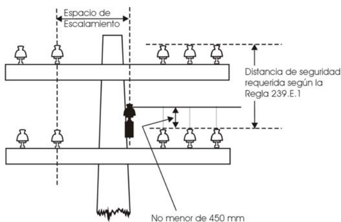
Figura 237-1 OBSTRUCCIÓN DEL ESPACIO DE TRABAJO POR CABALLETE
