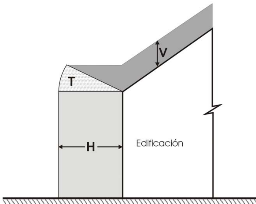
Figura 234-1(C) DISTANCIA DE SEGURIDAD TRANSICIONAL CUANDO "H" ES MAYOR QUE "V"
