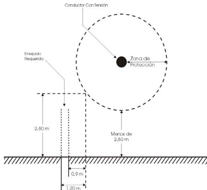
Figura 124-2 ENREJADO UTILIZADO COMO GUARDAS
