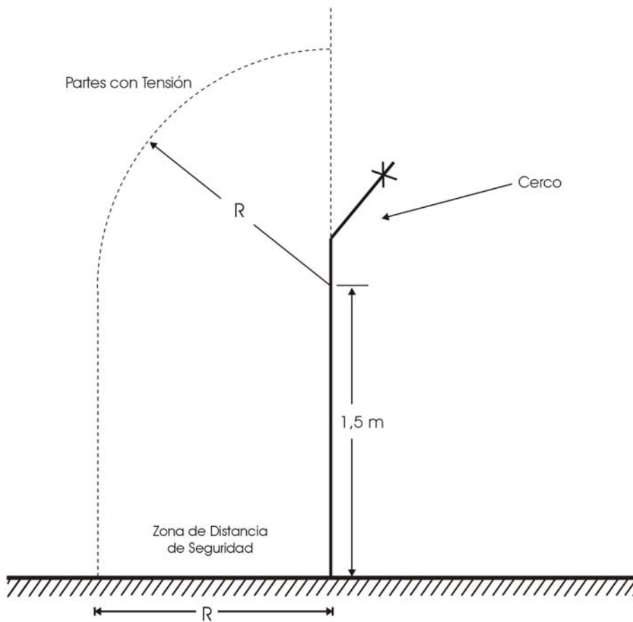
Figura 110-1 DISTANCIA DE SEGURIDAD PARA LOS CERCOS DE LA PLANTA DE SUMINISTRO ELÉCTRICO
