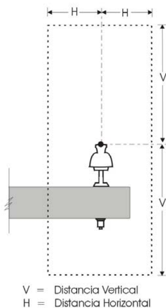
Figura 235-1 Diagrama de distancia para un conductor energizado
