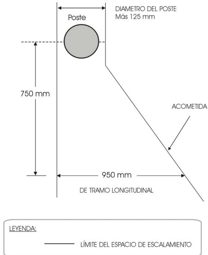
Figura 236-1 REGLA 236G, EXCEPCIÓN 3
