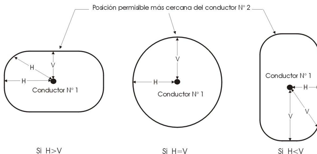
Figura 233-3 RECUBRIMIENTO DE LA DISTANCIA DE SEGURIDAD
